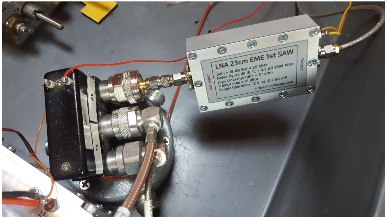
Neuer 23cm-LNA bei DH5YM
