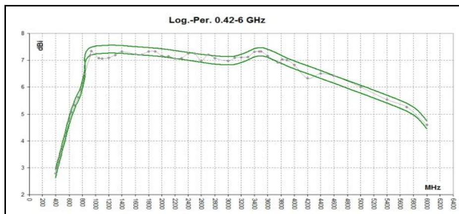
Breitbanderreger 420MHz bis 6GHz ( https://www.tgn-technology-online.com )
