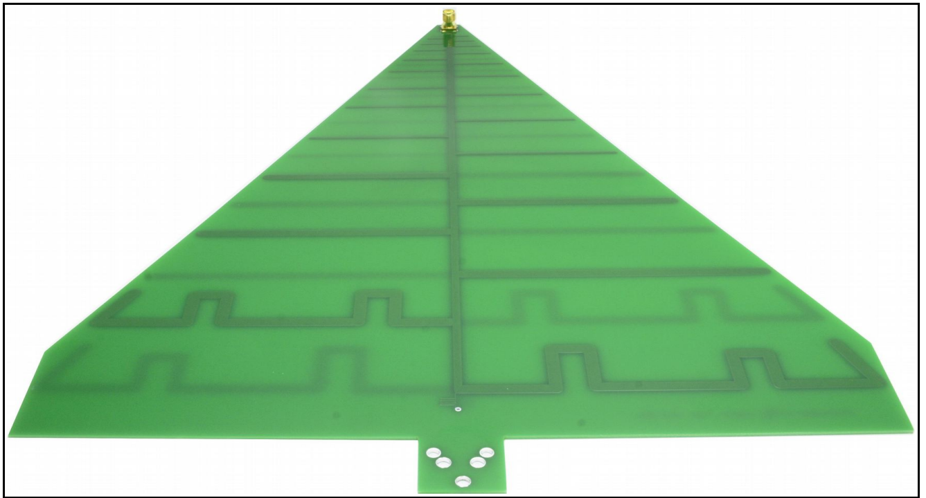
Breitbanderreger 420MHz bis 6GHz ( https://www.tgn-technology-online.com )
